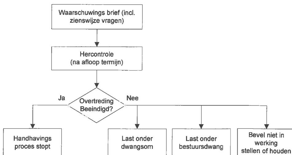
Schema reactie 2
